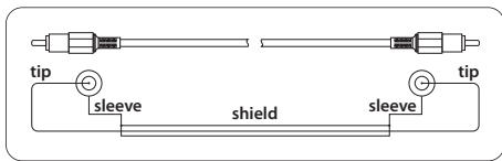
Fig. 5.1: RCA cable
